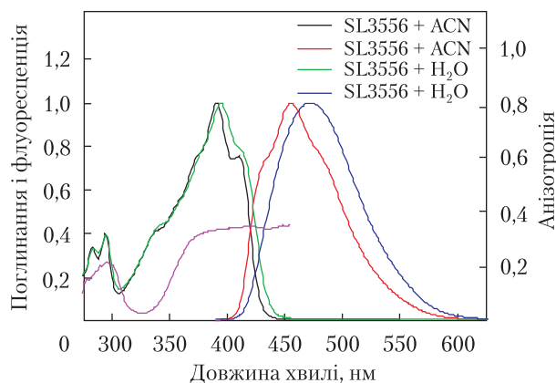
Рис. 3. Нормалізовані лінійні спектри поглинання і випромінювання барвника 3 в АЦН та воді (чорний – поглинання барвника 3 в АЦН, червоний – флуоресцентної барвника 3 в АЦН, зелений – поглинання барвника 3 у воді, синій – флуоресценція барвника 3 у воді, рожевий – анізотропія)
