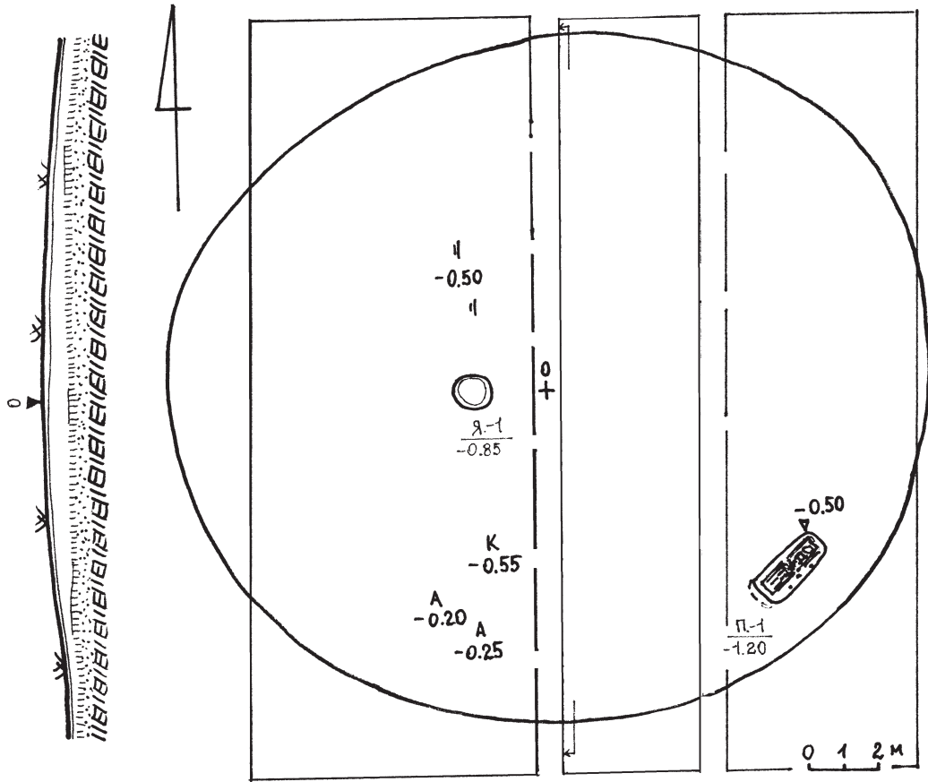
Рис. 1. Волошине, с., група II, курган № 2. План і профіль центральної бровки
