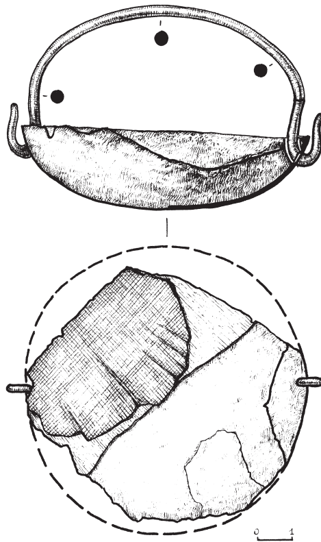
Рис. 8. Сегментоподібна чаша: Залізо. Схема розташування відбитків текстилю та шкіри на дні
