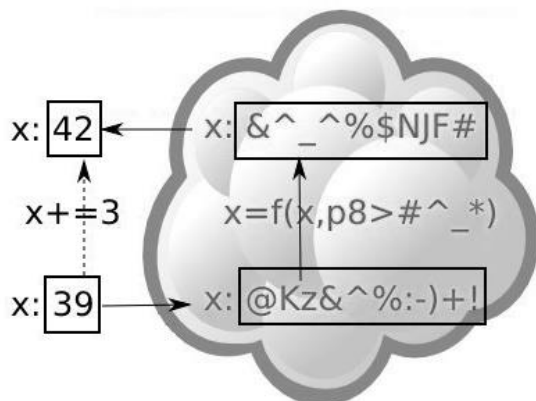
Рис. 4. Повністю гомоморфне шифрування в хмарних базах даних без знання вмістимого запиту повідомлення
