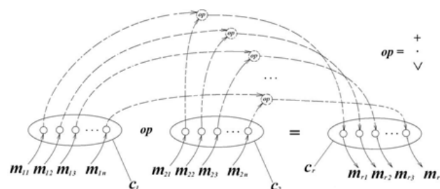
Рис. 2. Виконання векторних операцій над пакетними шифротекстами гомоморфного шифрування
