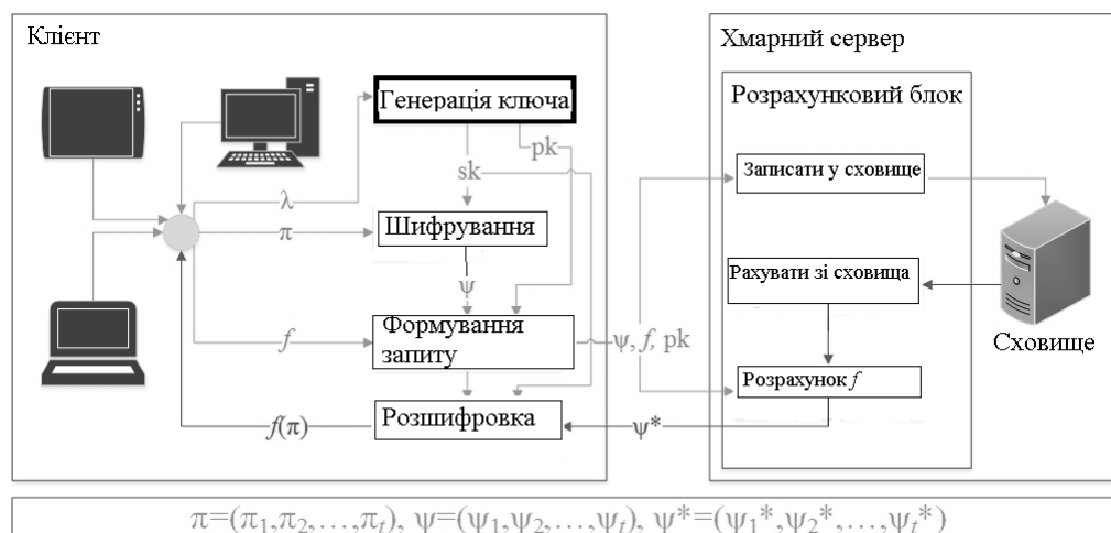
Рис. 1. Алгоритм безпечних хмарних обчислень над зашифрованими даними
