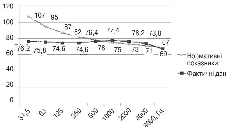
Рівень звукового тиску (дБ) в октавних смугах з середньогометричними частотами (Гц) на ліній розливу у металеву тару
