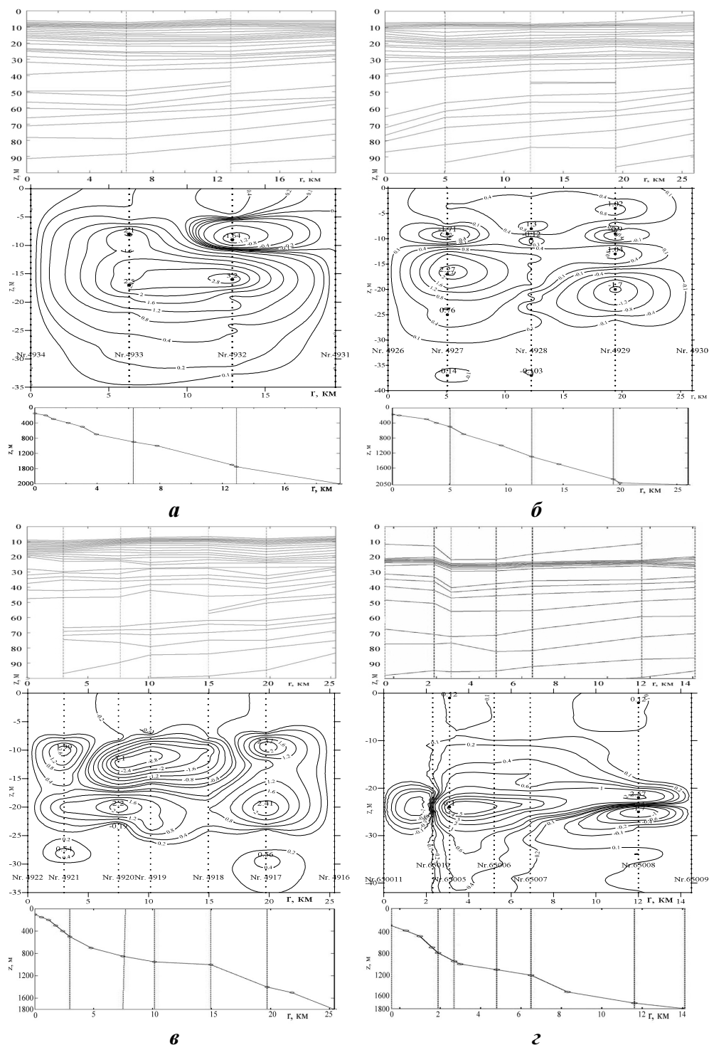
Р и с . 2 . Изолинии поля (вверху), аномалии поля температуры в разрезе ОЧТ (посередине), профиль дна (внизу): НИС «Проф. Колесников», рейс 27-2, 8 июля 1991 г., ст.4931 – 4934 (а), ст.4926 – 4930 (б), ст.4916 – 4922 (в), НИС «Трепанг», рейс 18, 12 октября 1997 г., ст.65011 – 65005 (з).
