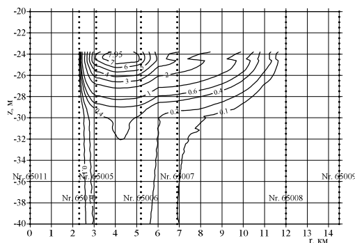
Рис. 12. Изолинии восстановленного поля аномалии температуры.
