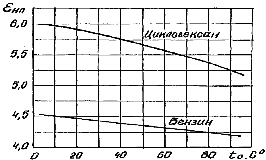
Рис.1. Вплив температури повітря на впуску на найвищий допустимий ступінь стиску [8]
