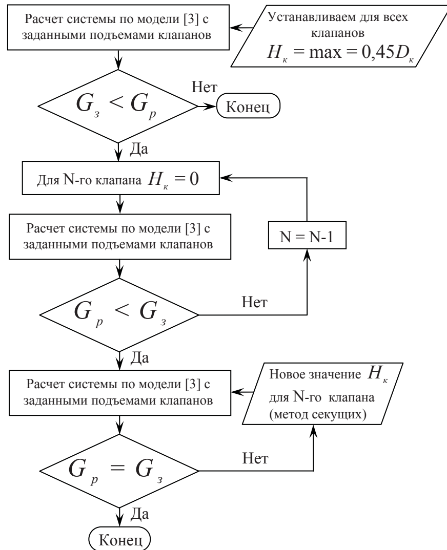
Рис. 2. Блок-схема первого варианта алгоритма, определяющего положения регулирующих клапанов для заданного расхода пара
