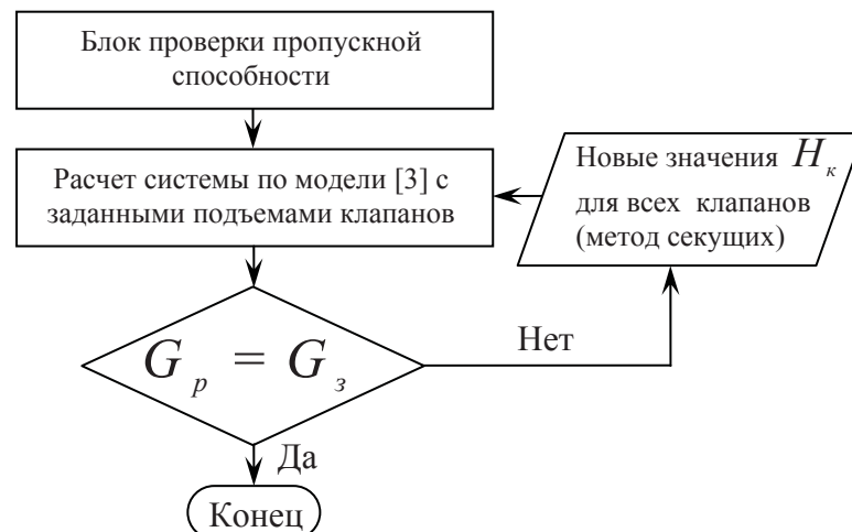
Рис. 3. Блок-схема 2-го и 3-го вариантов алгоритма, определяющего положения регулирующих клапанов для заданного расхода пара
