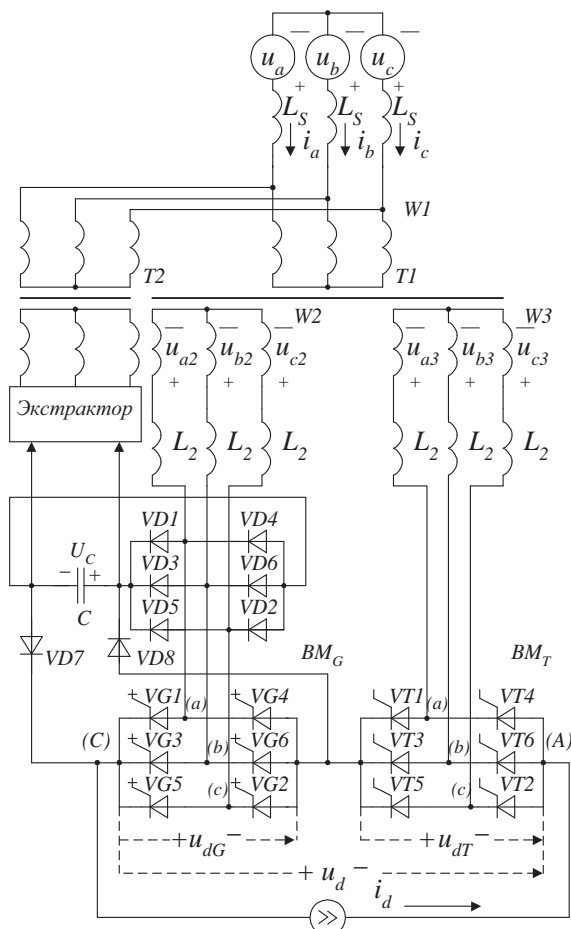
Рис. 1. Схема двенадцатипульсного КУВ
