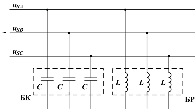
Рис. 5. Подключение к сети трехфазных батарей конденсаторов и реакторов
