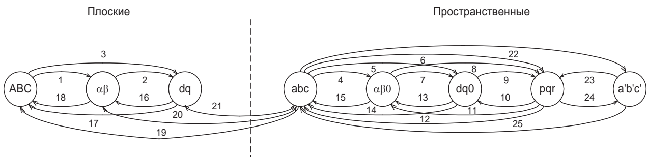
Рис. 6. Возможные преобразования координат
