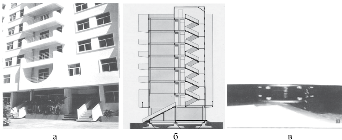
Рис.1. Здание, оснащенное виброизоляционной системой резиновых опор: (а – внешний вид здания; б – схематическое изображение; в – внешний вид резиновой опоры)
