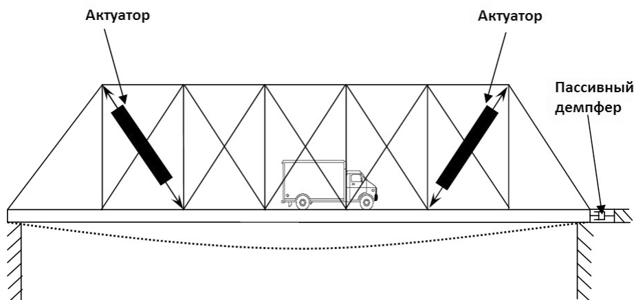
Рис. 7. Пример использования гибридной системы управления вибрациями
