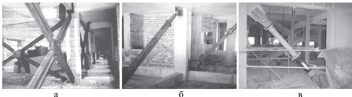
Рис. 4. Виды демпферов
