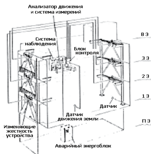
Рис.6. Фотографический снимок и схема здания, оснащенного полуактивной защитой от землетрясений с помощью переменной жесткости строительных элементов
