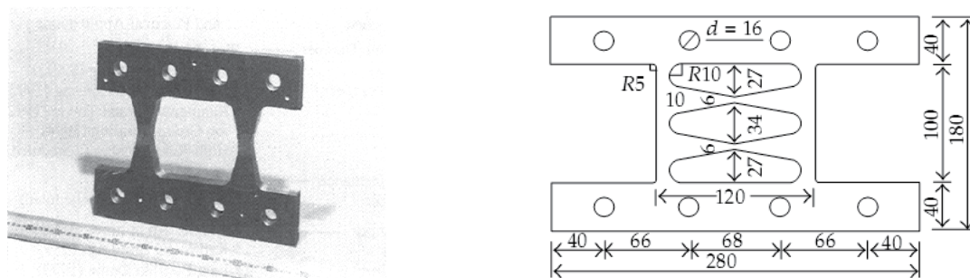
Рис.2. Различные типы металлических демпферов [1, 4].
