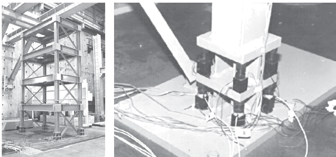
Рис. 8. Строительная модель с закрепленными на ней пьезоэлектрическими актуаторами
