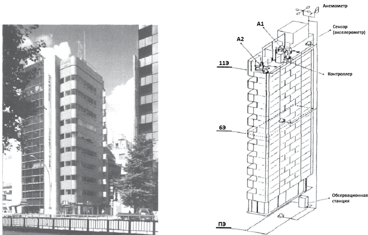
Рис. 5. Фотографический снимок и схематическое изображение здания, оснащенного схемой активного управления вибрациями
