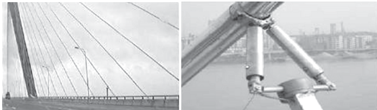
Рис. 9. Мост с магнитоэлектрическими актуаторами
