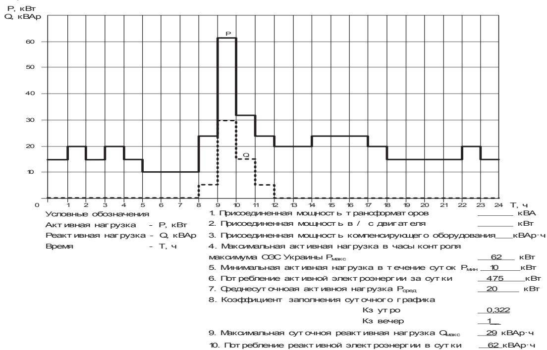
Рис. 7, а. Суточный график летнего периода
