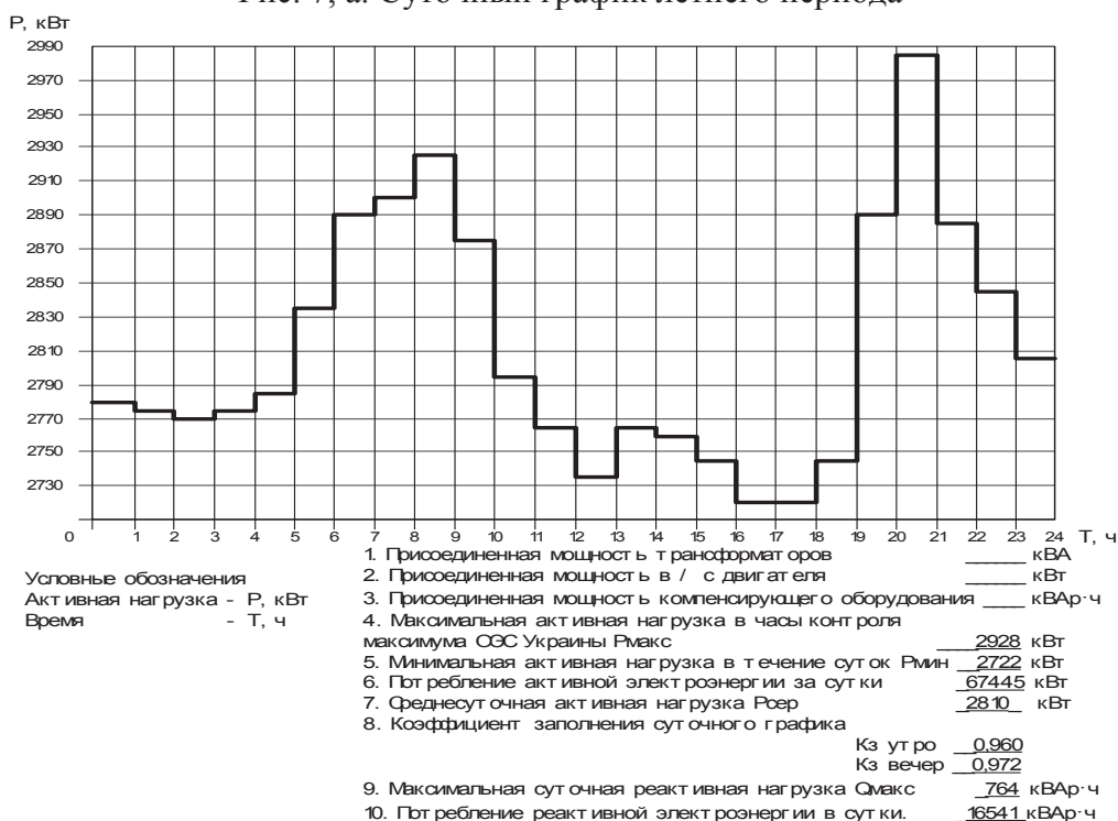
Рис. 7, б. Суточный график зимнего периода
