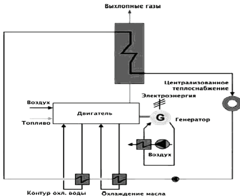
Рис. 2. Принципиальная схема газопоршневой когенерационной установки
