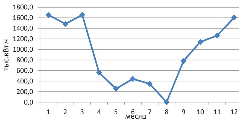
Рис.10. Динамика потребления электроэнергии
