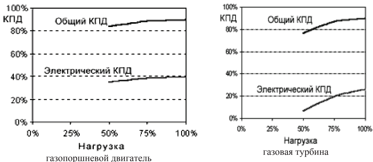
Рис. 1. Графики зависимости КПД от нагрузки
