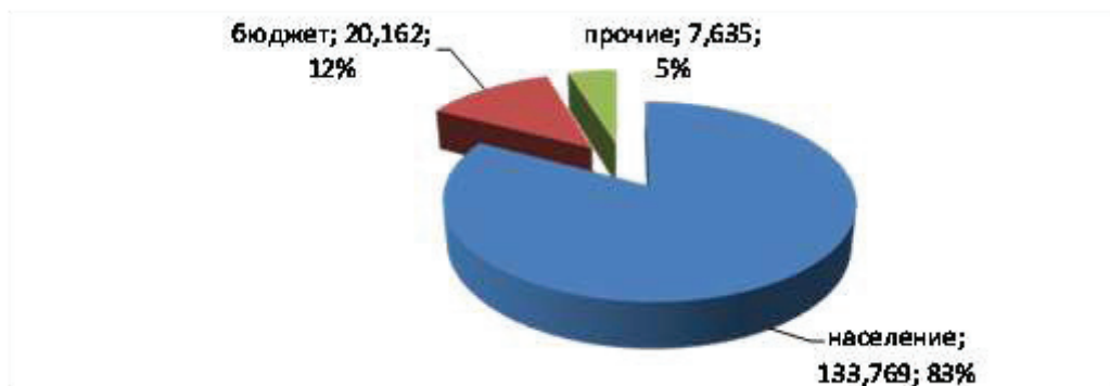
Рис. 4. Структура нагрузки по отоплению и вентиляции
