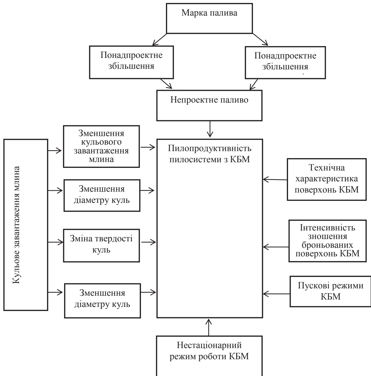
Рис. 1. Блок-схема впливу різних факторів на ефективність роботи КБМ пілопродуктивності пілосистем котлів при спалюванні непроекних видів палива
