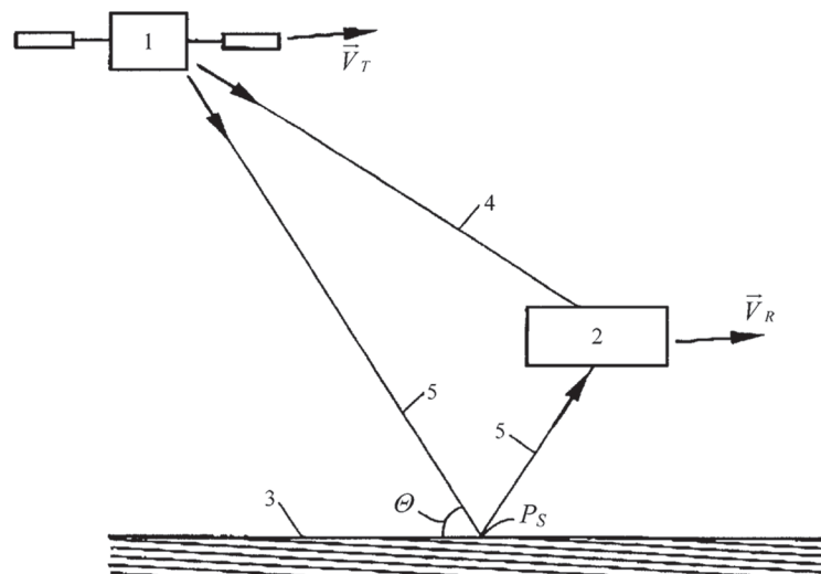
Рис. 1. Схема роботи системи моніторингу рівня води водойми:
