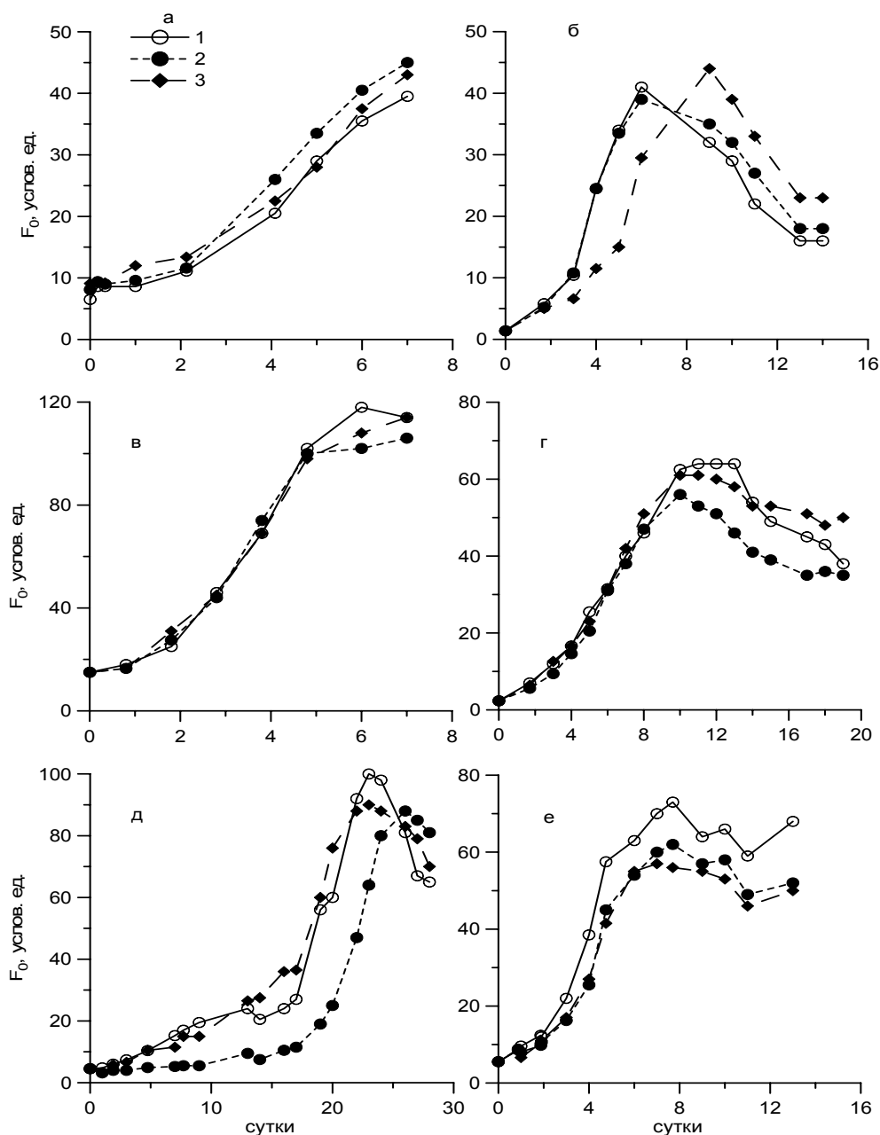
Рис. 1. Рост динофитовых водорослей на нитратах (1), аммонии (2) и мочеvine (3): G. fissum (а – 19 \mu\text{Э} \times \text{м}^{-2} \times \text{с}^{-1} , б – 105 \mu\text{Э} \times \text{м}^{-2} \times \text{с}^{-1} ), P. cordatum (в – 19 \mu\text{Э} \times \text{м}^{-2} \times \text{с}^{-1} , г – 105 \mu\text{Э} \times \text{м}^{-2} \times \text{с}^{-1} ), H. triquetra (д – 19 \mu\text{Э} \times \text{м}^{-2} \times \text{с}^{-1} , е – 105 \mu\text{Э} \times \text{м}^{-2} \times \text{с}^{-1} )
