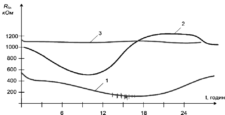
Рис. 3 Добові зміни активного опору ізоляції: 1-весна, осінь; 2-літо; 3-зима
