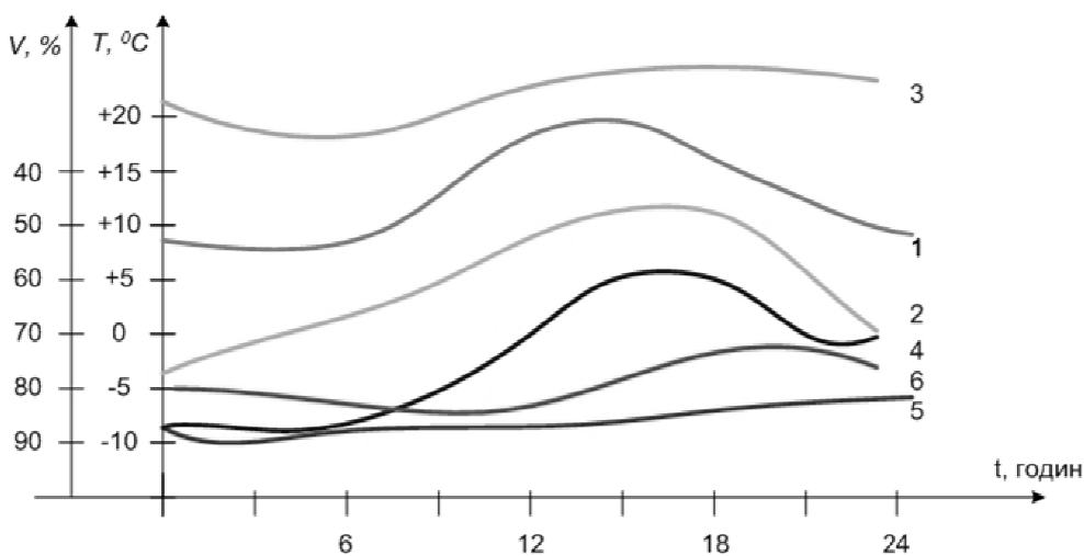
Рис. 4 Добові зміни температури T °С і відносної вологості V %
