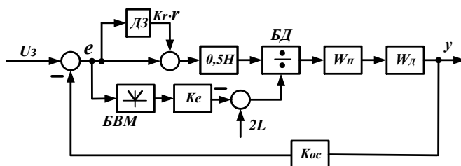
Рисунок 2 – замкнута система керування
