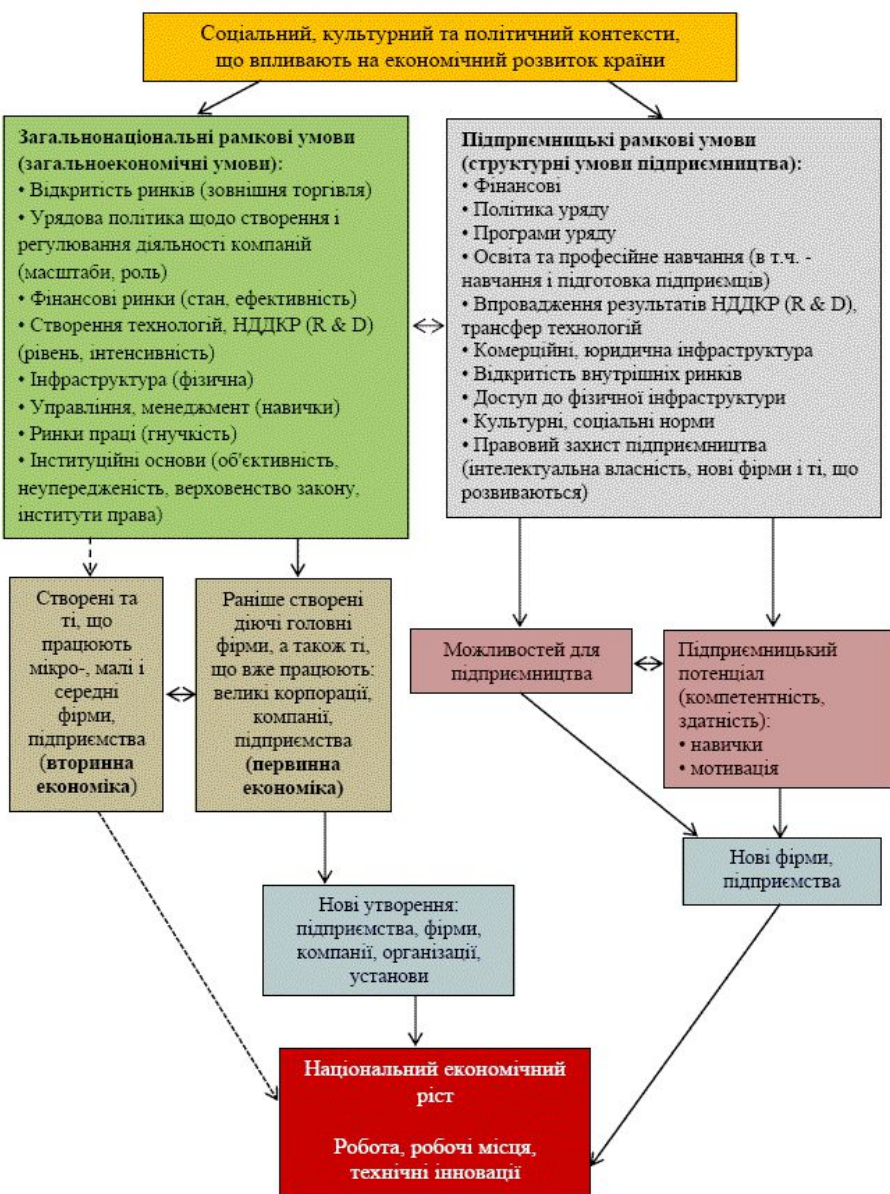
Рис. 1. Концептуальна модель національного економічного росту (за GEM, 2004)
