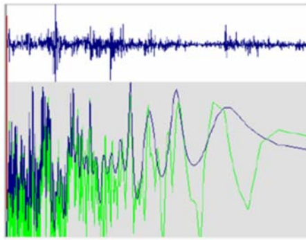
Рис. 4. Оцінка максимальної ентропії для UX
