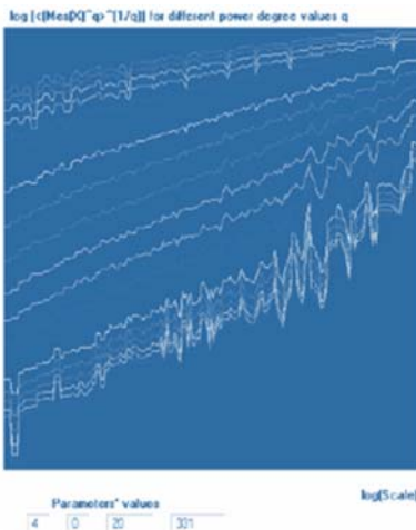
Рис. 5. Мультифрактальний спектр сингулярності індексу ПФТС
