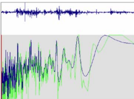
Рис. 3. Оцінка максимальної ентропії для ПФТС
