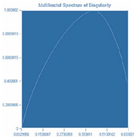
Рис. 6. Мультифрактальний спектр сингулярності індексу UX
