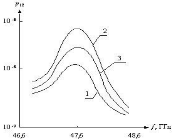
Рис. 1. Залежність вірогідності утворення вільних радикальних пар p_{12} для насіння гороху від частоти зовнішнього ЕМВ при t=10 хв.: 1 – P=5 мкВт/см 2 ; 2 – P=12 мкВт/см 2 ; 3 – P=20 мкВт/см 2
