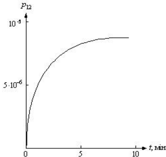
Рис. 2. Залежність вірогідності утворення вільних радикальних пар p_{12} в насінні гороху від часу дії зовнішньої ЕМВ при P=10 мкВт/см 2 , f=47,6 ГГц
