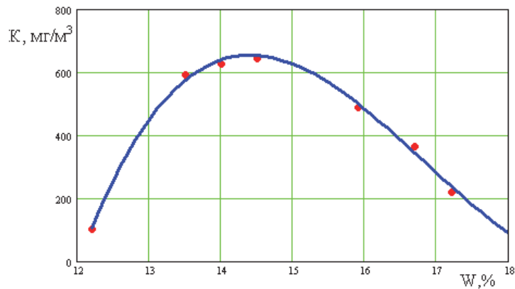
Рис. 1. Залежність концентрації озону в зерновій масі залежно від її вологості: • – дані отримані за матеріалами досліджень; — – графік функції побудований за емпіричною формулою
