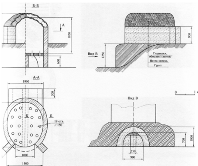
Мал. 6. Гончарне горно. Кульчин. Волинь. ХІХ–ХХ століття. За Наталією Кубицькою [Кубицька, 2004, с. 51].
