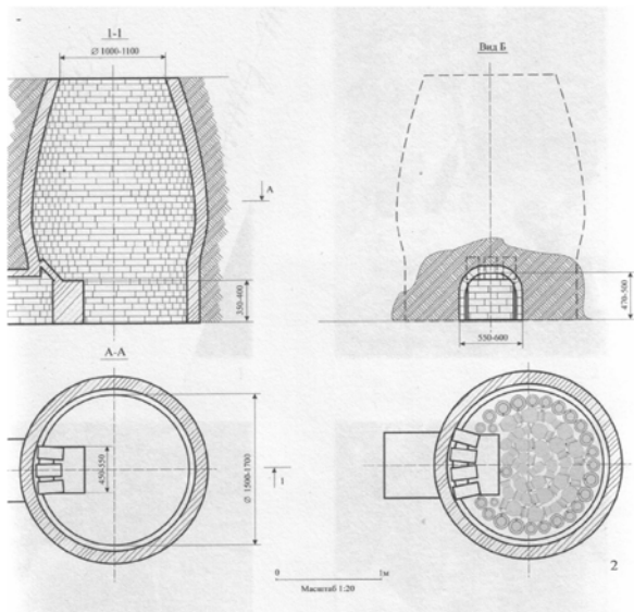
Мал. 8. Гончарне горно. 1 – загальний вигляд; 2 – спосіб укладання глиняних виробів для випалювання. Рокита. Волинь. XIX–XX століття. За Наталією Кубицькою [Кубицька, 2006, с. 216, 218].
