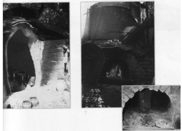
Мал. 5. Гончарне горно. Кульчин. Волинь. ХІХ–ХХ століття. За Наталією Кубицькою [Кубицька, 2004, с. 51].
