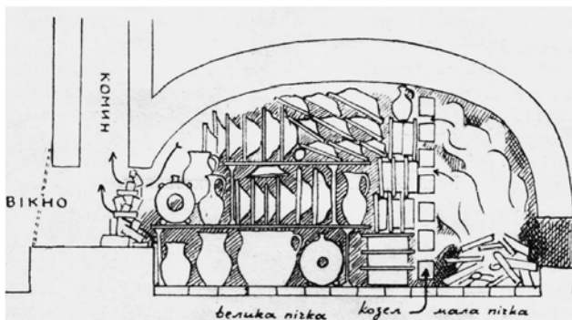
Мал. 3. Випалювальна споруда. Гуцульщина. XIX–XX століття. За Юрієм Лащуком [Лащук, 1956, с. 37].
