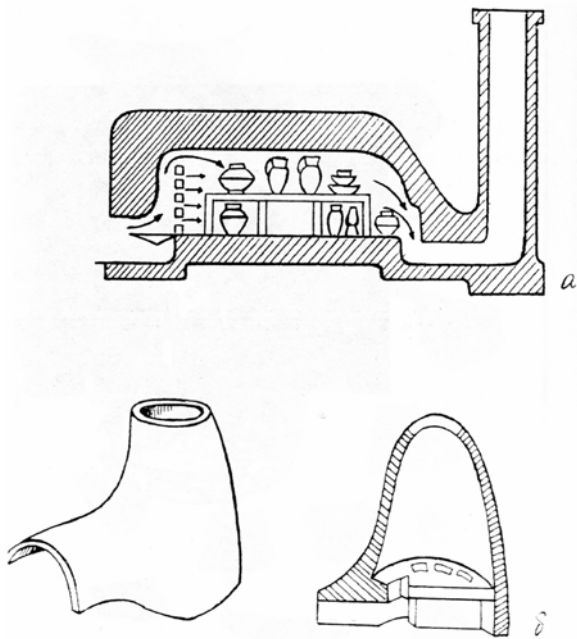
Мал. 4. Випалювальні споруди; а – "лежаче" горно; б – гончарна піч. Пістинь. Івано-Франківщина. ХІХ–ХХ століття. За Олегом Слободян [Слободян, 2001, с. 90].
