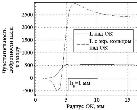
Рис. 2. Зависимость чувствительности добротности п.к.к. к изменению зазора от радиуса ОК ( h_B – зазор между ВТП и ОК)
