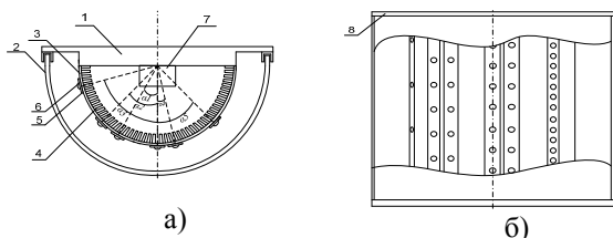
Рисунок 2 – Конструкція світлодіодного світильника: а – вид спереду; б – вид знизу; 1 – підставка основи; 2 – оптично прозора кришка; 3 – профіль світильника; 4 – радіаторні решітки; 5 – світлодіодна лінійка; 6 – світлодіод; 7 – блок живлення; 8 – торцева кришка
