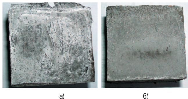
Рисунок 2 – Зовнішній вид зразка бетону на основі зололужного цементу з вмістом пластифікуючої добавки: а) – 1,5 %; б) – 0,05 %
