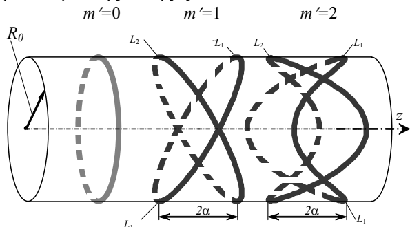
Рис. 1. Расположение селекционирующих контуров на общей цилиндрической поверхности
