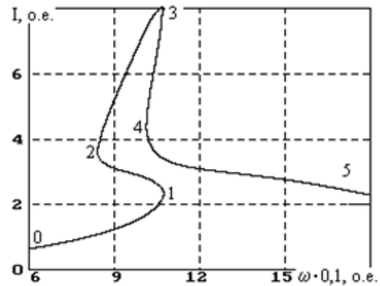
Рис. 4. Амплитудочастотная характеристика последовательной феррорезонансной цепи
