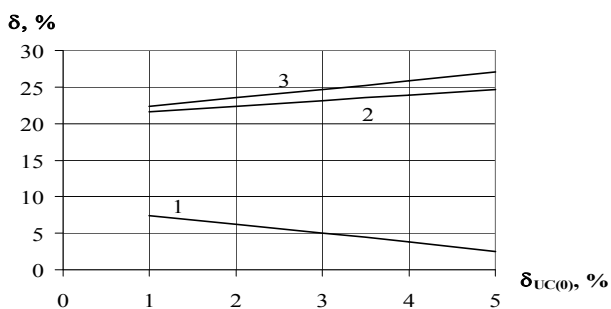
Рис. 5. Зависимость допусков в разрядной цепи для набора допусков параметров импульса вида:
