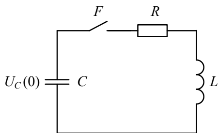
Рис. 1. Эквивалентная схема разряда ВИИУ. U_C(0) , C , L , R , – зарядное напряжение конденсатора, емкость конденсатора, индуктивность разрядной цепи, активное сопротивление разрядной цепи; F – коммутатор
