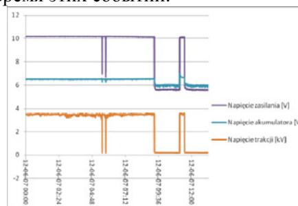
Рис. 6. Регистрация питающих напряжений 07.06.
