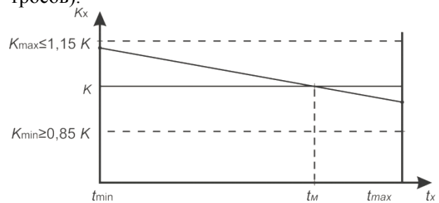
Рис. 4. Зависимость натяжения компенсированного контактного провода от температуры у средней анкеровки: t_m – температура, при которой струны располагались вертикально
