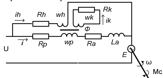
Рис. 6. Електрична схема заміщення двигуна постійного струму змішаного збудження
