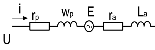
Рис. 1. Електрична схема заміщення двигуна послідовного збудження
