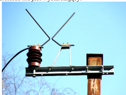
Rys. 2. Nieprawidłowe rozstawienie elektrod wyładowczych w odgromniku różkowym
