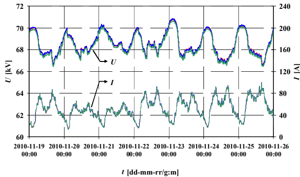
Рис. 5. Сравнение изменений фазовых напряжений на шинах 110 кВ и токов нагрузки в период измерения
