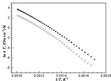
Рис. 9. Температурні залежності загальної провідності (об'ємної + зернограничної) електролітів 10Sc1CeSZ: Δ — DKKK; ■ — ППМ.
