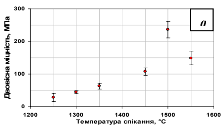
Рис. 7. Залежність двовісної міцності ОП кераміки ППМ від температури спікання (а) та поверхня руйнування (СЕМ) зразку, спеченого при 1550 °С (б).
