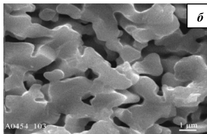
Рис. 7. Залежність двовісної міцності ОП кераміки ППМ від температури спікання (а) та поверхня руйнування (СЕМ) зразку, спеченого при 1550 °С (б).
