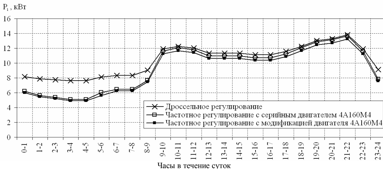
Рис.1. Потребление активной мощности электроприводом насоса при различных способах регулирования
