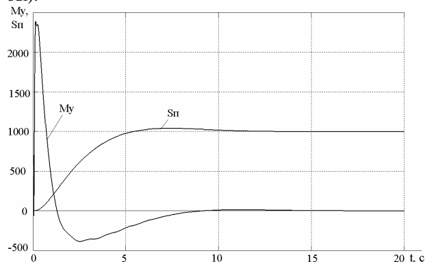
Рис.4. Графики изменения момента M_y и перемещения рабочего органа S_{п} системы с ПИД-регулятором момента и ФР положения
