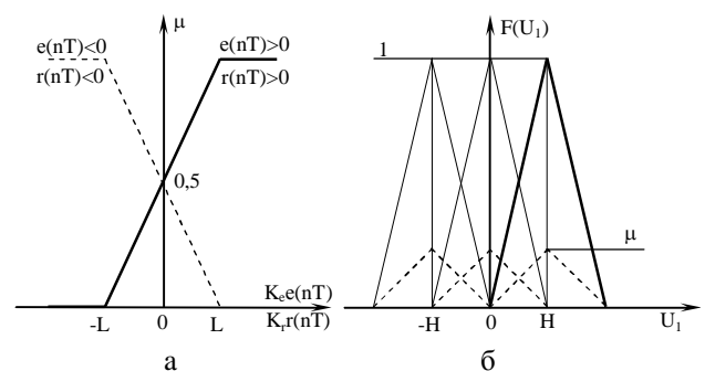
Рис.3. Функции принадлежности входного (а) и выходного (б) сигналов фаззи-регулятора
