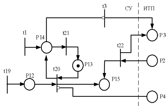
Рис.2. Модель тягового электротехнического комплекса с защитой от срыва коммутации
