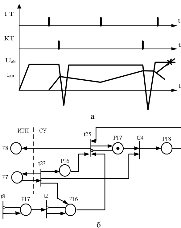
Рис.3. Временные диаграммы (а) и модель тягового комплекса с защитой от срыва коммутации при ложном импульсе (б)
