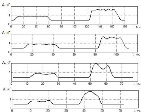
Рис. 15. Графики взвешивания модели автомобиля в динамике
