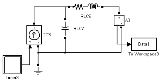
Рис. 6. RLC- модель 2-го порядка
