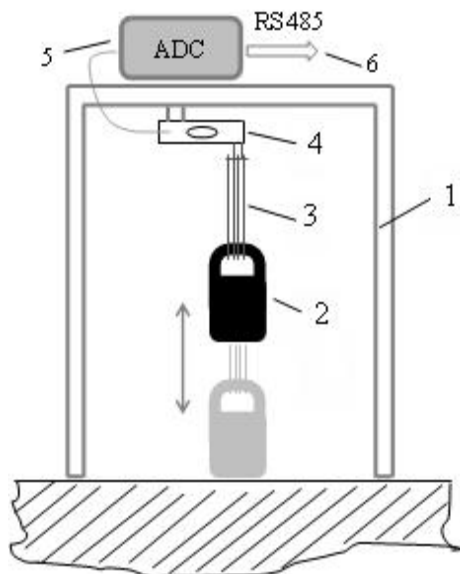
Рис. 10. Экспериментальный стенд для определения массы колеблющегося груза: 1 – рама; 2 – гиря; 3 – резиновый подвес; 4 – тензометрический датчик; 5 – аналогово-цифровой блок; 6 – последовательный интерфейс
