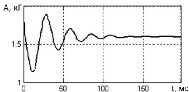
Рис. 12. Сигнал, полученный с тензометрического датчика
