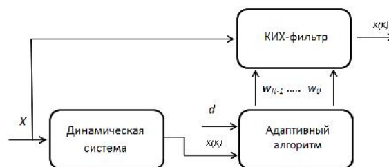
Рис. 4. Структурная схема адаптивной идентификации систем
