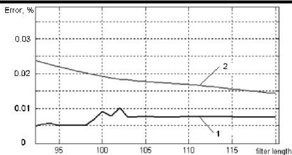
Рис. 13. Относительная погрешность обработки данных:
