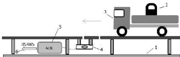
Рис. 14. Экспериментальный стенд для определения массы катящегося объекта:
