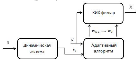
Рис. 5. Структурная схема получения результата методом адаптивной идентификации
