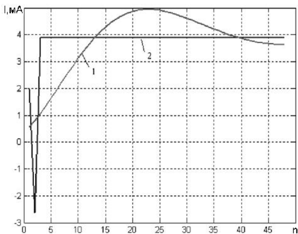
Рис. 7. График зависимости тока в модели от номера выборки: 1 – измеренное значение, 2 – результат обработки методом адаптивной идентификации (порядок алгоритма N=3 )
