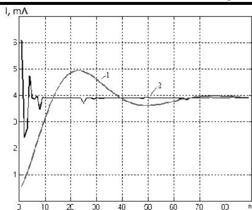
Рис. 9. График зависимости тока в модели от номера выборки: 1 – измеренное значение, 2 – результат обработки (порядок алгоритма N=12 )
