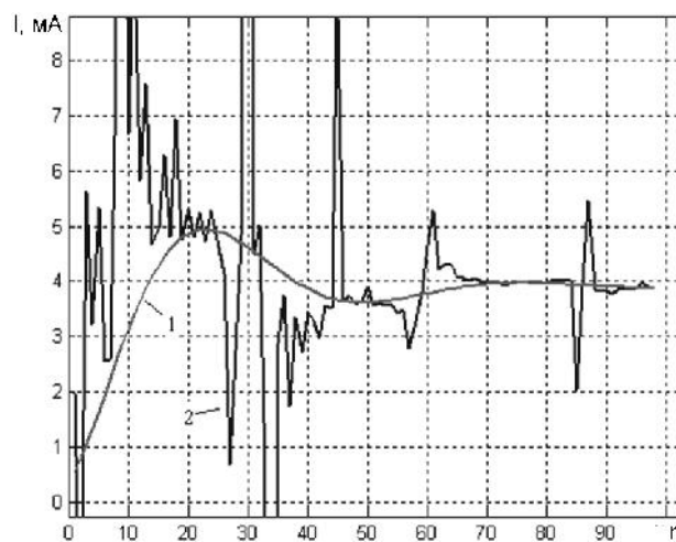
Рис. 8. График зависимости тока в модели от номера выборки: 1 – измеренное значение, 2 – результат обработки (порядок алгоритма N=3 )
