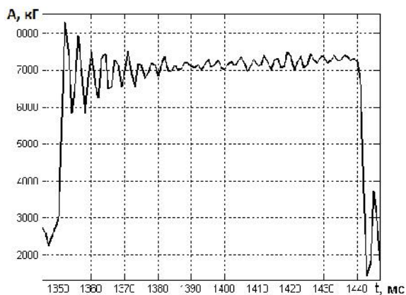
Рис. 1. Сигнал тензометрического датчика при наезде оси вагона на платформу весов
