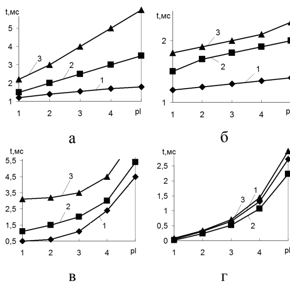
Рис. 3. Оценка времени выполнения операции при 1 - k = 1; 2 - k = 2; 3 - k = 3 : а – тип связи «1-M», EXISTS и IN, select ; б – тип связи «1-1», EXISTS и IN, select ; в – тип связи «1-1», Native, select ; г – тип связи «1-1», Native, update
