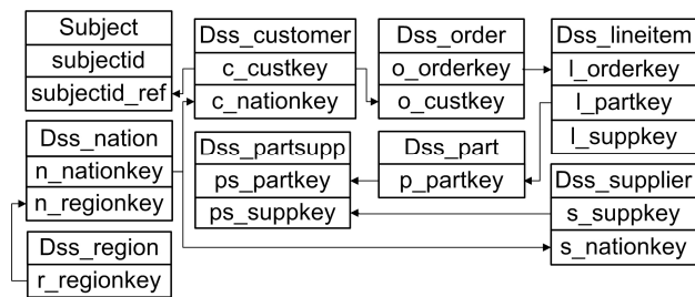
Рис. 7. Реляционная модель БД теста TPC-D
