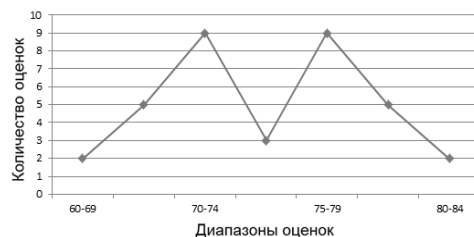
Рис. 8. Функция, характеризующая студента 3, набравшего за рассматриваемый период обучения одинаковое количество «хороших» и «удовлетворительных» баллов
