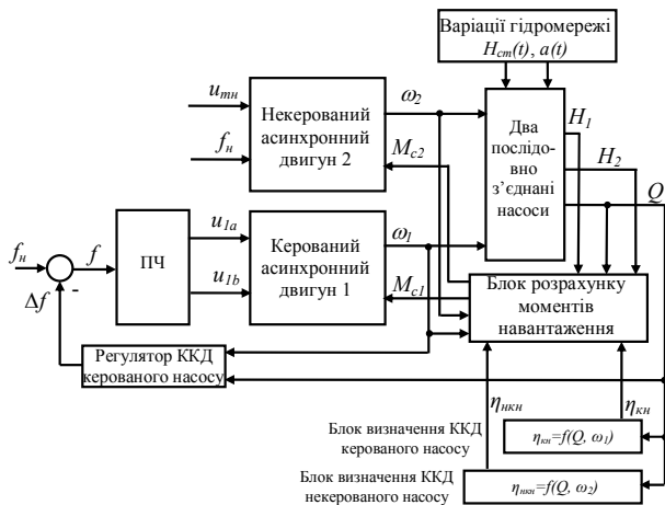
Рис. 1. Структурна схема системи керування
