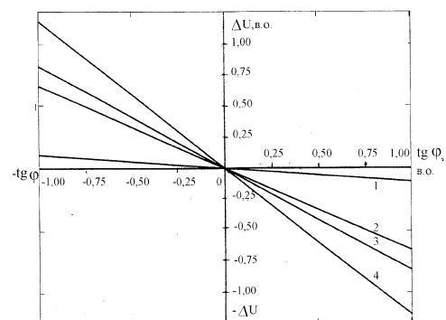
Рис.4. Залежність \Delta U^* = f(\text{tg} \varphi_D) :
