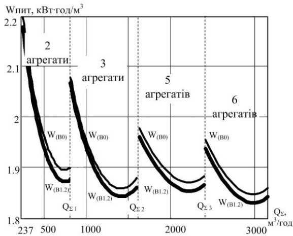
Рис. 7. Питомі витрати електроенергії ЕТК
