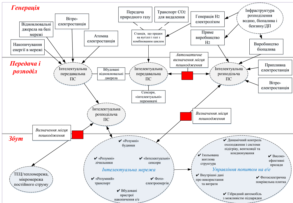
Рисунок 3 – Електроенергетика на базі концепції Smart grid
