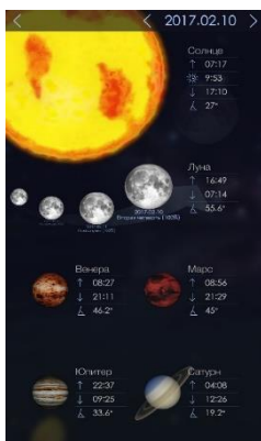
Рис. 2. Функція Sky Live
