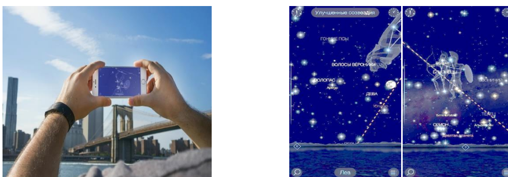
Рис. 1. Додаток Star Walk 2
