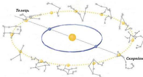
Рис. 6. Кульмінація сузір'я Скорпіона
