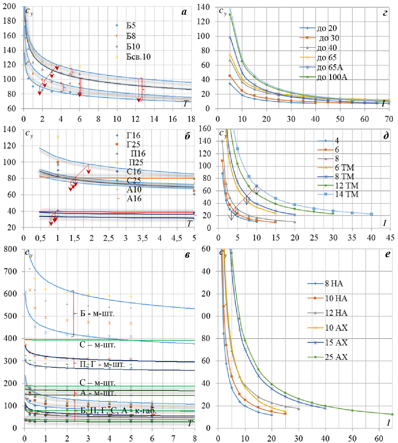
Рис. 2. Зависимости между продолжительностью ( T ) работы башенных ( a ) и стреловых мобильных ( b ) кранов на объекте, и удельной себестоимостью ( c_y ) механизированного монтажного процесса (для соответственного типоразмера), в том числе при различной крупности монтажных элементов ( b ); а также между сменной интенсивностью ( I ) бетонирования на объекте, и удельной себестоимостью ( c_y ) прицепных и автобетононасосов ( c ), торкрет-установок и торкрет-машин ( d ), установок и машин (машины с манипуляторами на автомобильном ходу) для набрызг-бетонирования ( e ).
