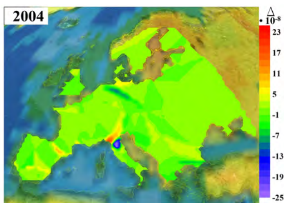
Рис. 7. Карта-схема розподілу швидкостей дилатації земної кори 10^{-8} 1/рік на території Європи у 2004 р.
