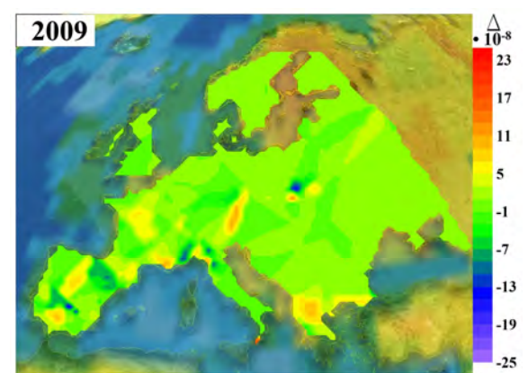
Рис. 9. Карта-схема розподілу швидкостей дилатації земної кори 10^{-8} 1/рік на території Європи у 2009 р.
