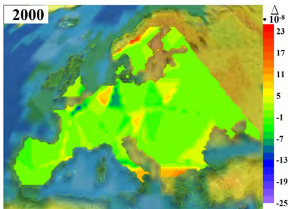
Рис. 6. Карта-схема розподілу швидкостей дилатації земної кори 10^{-8} 1/рік на території Європи у 2000 р.
