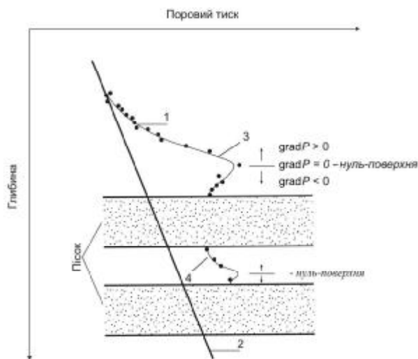
Рис. 2. Залежність порового тиску від глибини в басейні Бофорта, Канада (за даними [14], з доповненнями). Тиск: 1 – розрахунковий, 2 – гідростатичний; 3 – профіцит тиску; 4 – дефіцит тиску; grad P – градієнт тиску
