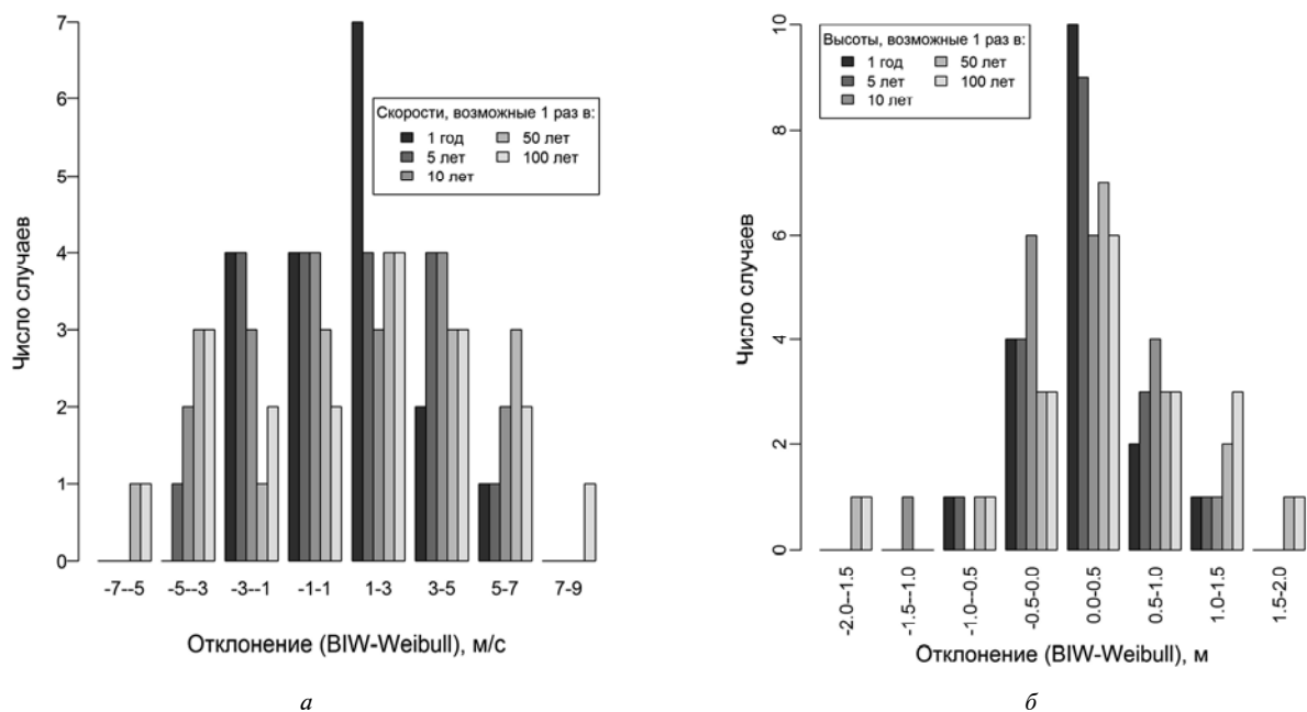
Рис. 4. Отклонение оценок вероятных скоростей ветра (а) и высот волн (б), вычисленных по моделям ВІW и Вейбулла (Weibull) для пунктов морской береговой сети Украины за период 1958–2012 гг.
