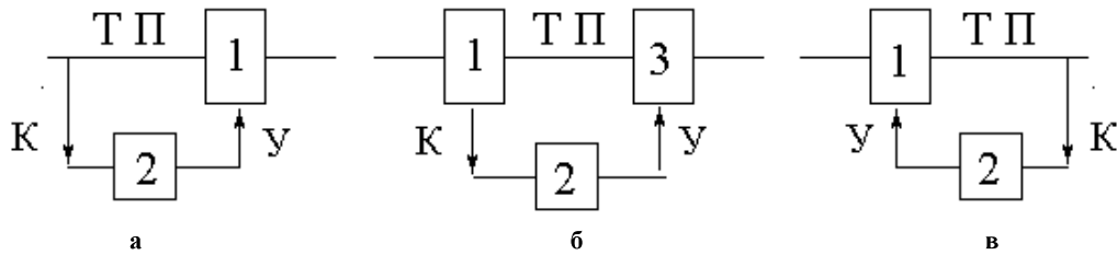
Рис. 2. Основні структури інформаційного забезпечення ТП: а – прямого зв'язку; б – посереднього та в – зворотного зв'язків
