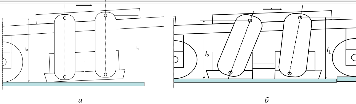
Рис. 2. Проходження односекційним (а) та двосекційним (б) магнітним блоком довантажувача нерівності рейкової колії
