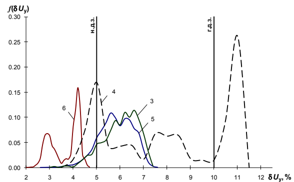
Рис. 6. Емпіричні розподіли відхилень напруги на шинах 10 кВ чотирьох різних підстанцій
