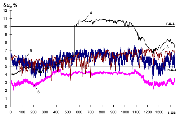
Рис. 5. Усталене відхилення напруги на шинах 10 кВ чотирьох різних підстанцій
