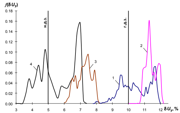
Рис. 2. Емпіричні розподіли відхилень напруги на шинах 110 кВ чотирьох різних підстанцій
