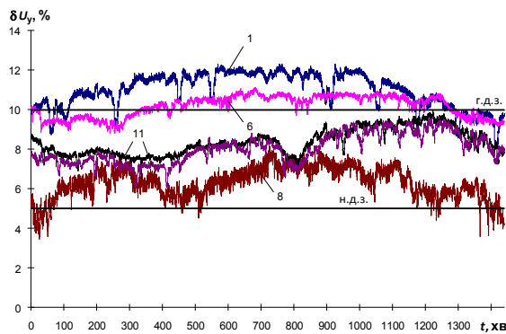
Рис. 3. Усталене відхилення напруги на шинах 35 кВ чотирьох різних підстанцій
