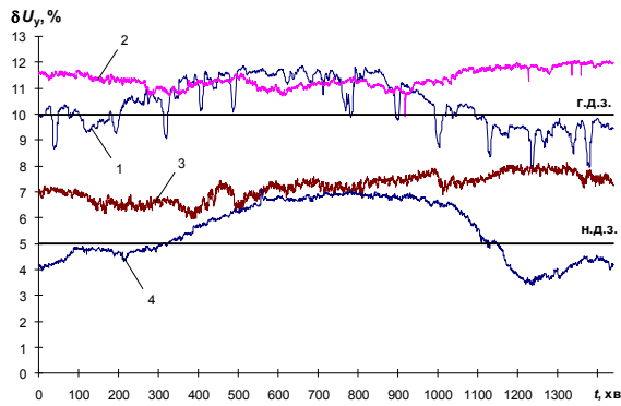
Рис. 1. Усталене відхилення напруги на шинах 110 кВ чотирьох різних підстанцій
