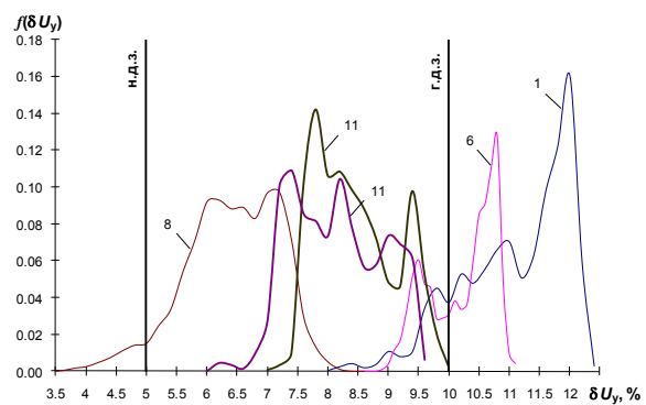
Рис. 4. Емпіричні розподіли відхилень напруги на шинах 35 кВ чотирьох різних підстанцій
